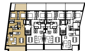
plan eerste verdieping
