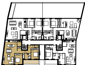
plan gelijkvloers
