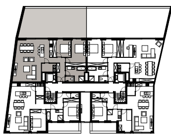
plan gelijkvloers
